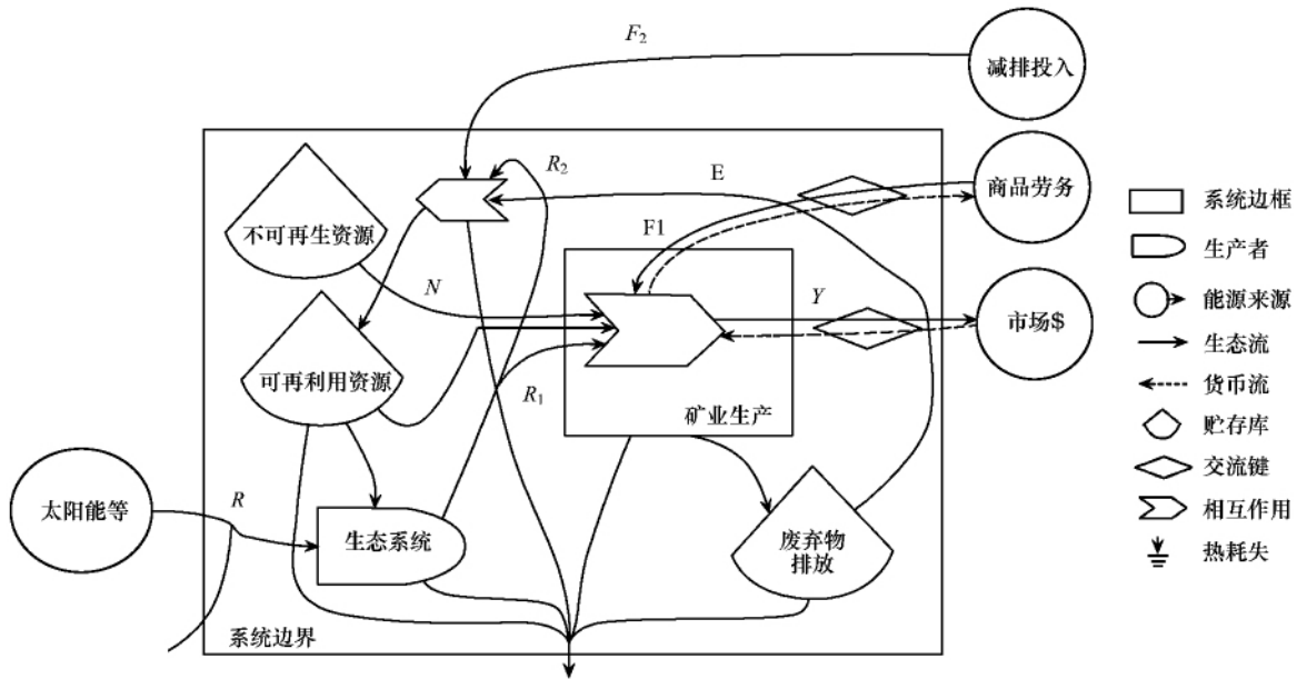
图 1 典型煤炭矿区物能流简图
